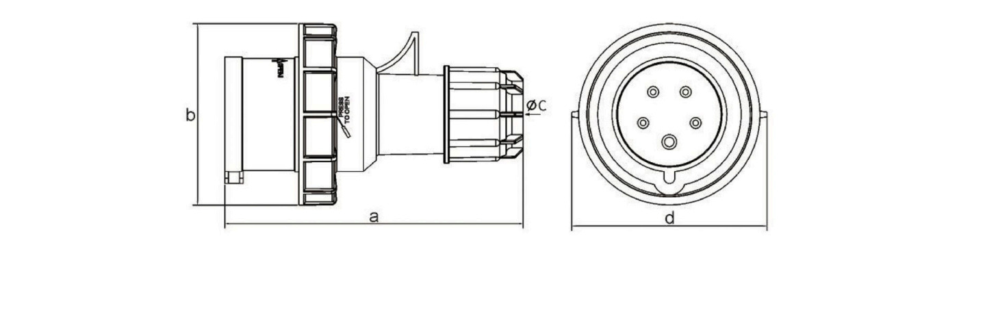
外型尺寸图 Dimensions
