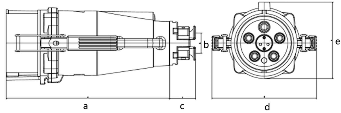
外型尺寸图 Dimensions
