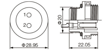
注 :M20×1.5 螺纹 Note :M20×1.5 thread
