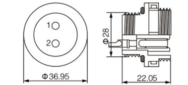
注 :M28×1.5 螺纹 Note :M28 x 1.5 thread
